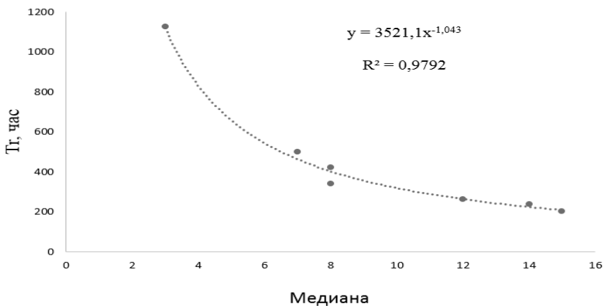
Рис. 6. Зависимость времени T_r от медианы в кластерах поселений Российской Федерации
