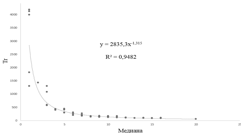
Рис. 1. Зависимость характеристики T_r от медианы (кружками обозначены эмпирические данные)
