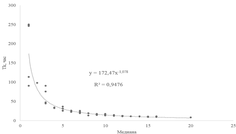
Рис. 2. Зависимость характеристики T_k от медианы (кружками обозначены эмпирические данные)
